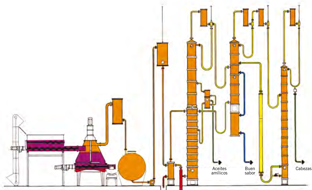
Instalacion de destilacion continua orujo o rectificacion de flemas.
